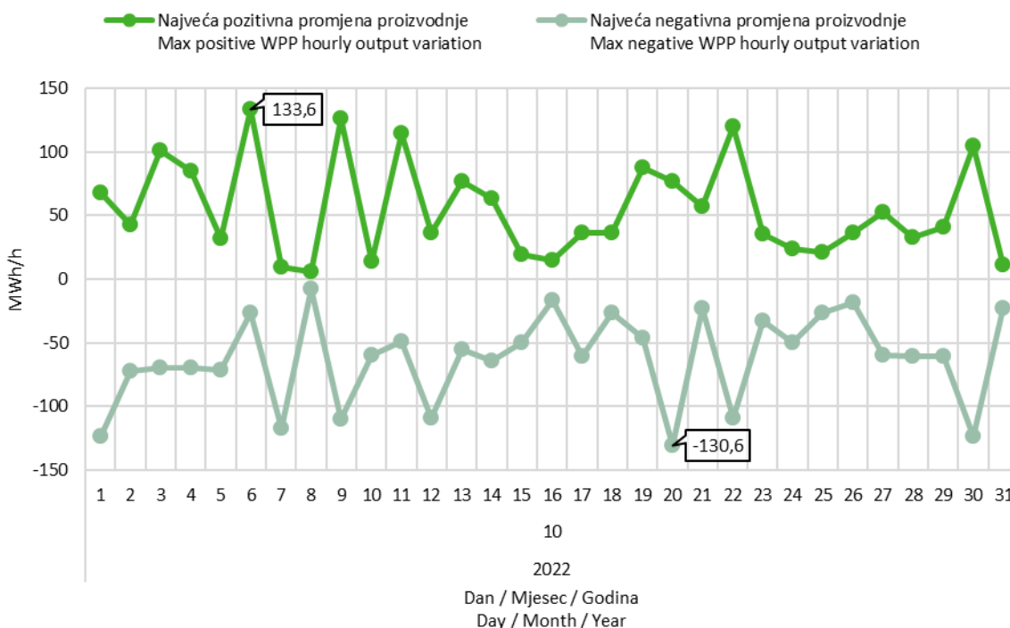
Slika 9 Maksimalna pozitivna i maksimalna negativna promjena satne proizvodnje VE u listopadu 2022. godine
