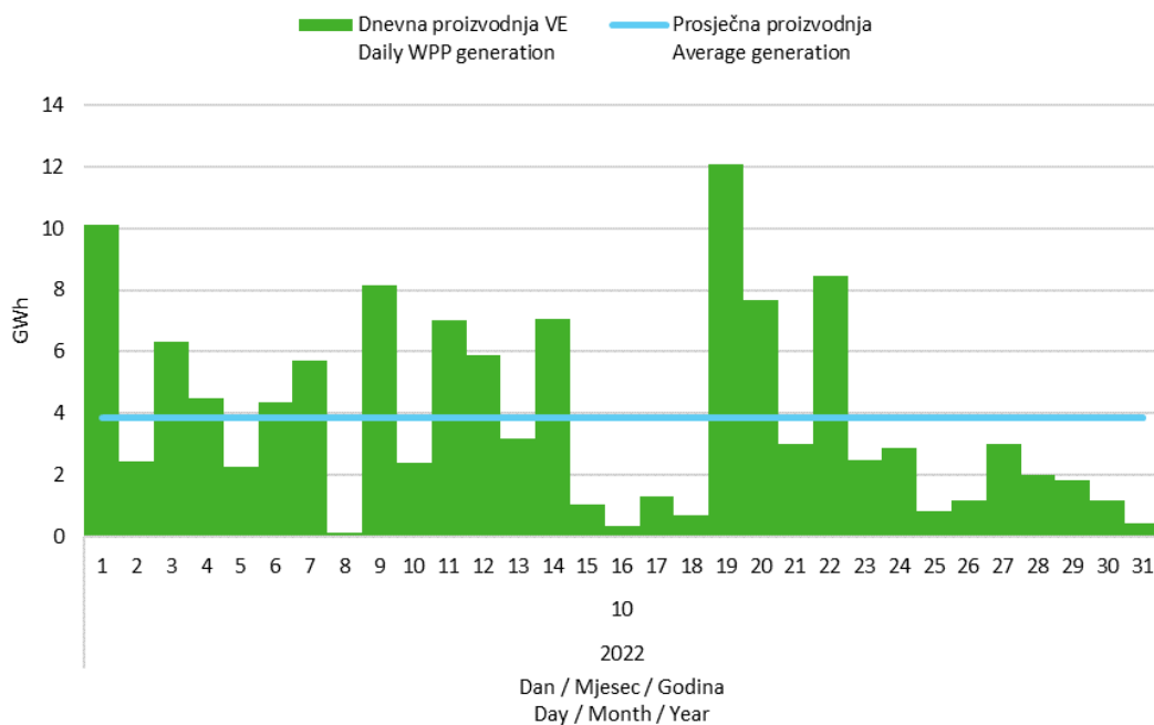
Slika 5 Dnevna proizvodnja svih vjetroelektrana u listopadu 2022. godine
