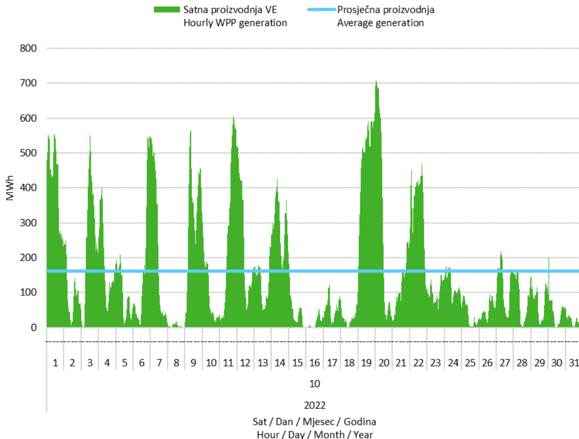
Slika 2 Satna proizvodnja svih vjetroelektrana u listopadu 2022. godine
