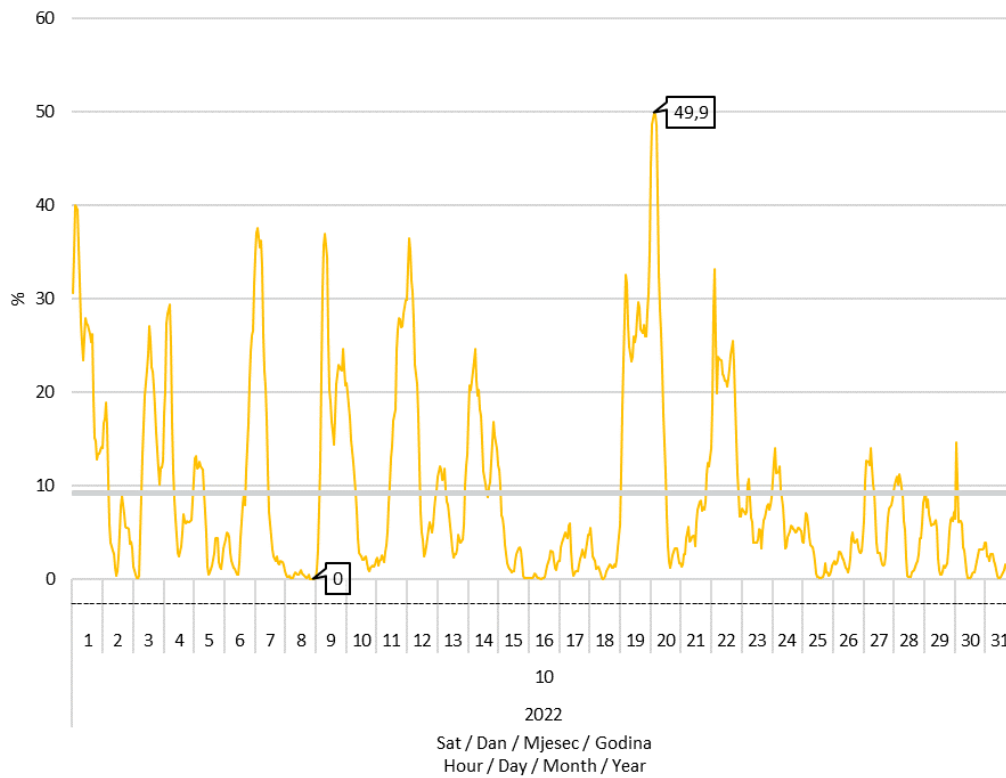
Slika 8 Udio proizvodnje vjetroelektrana u pokrivanju satnog opterećenja elektroenergetskog sustava u listopadu 2022. godine
