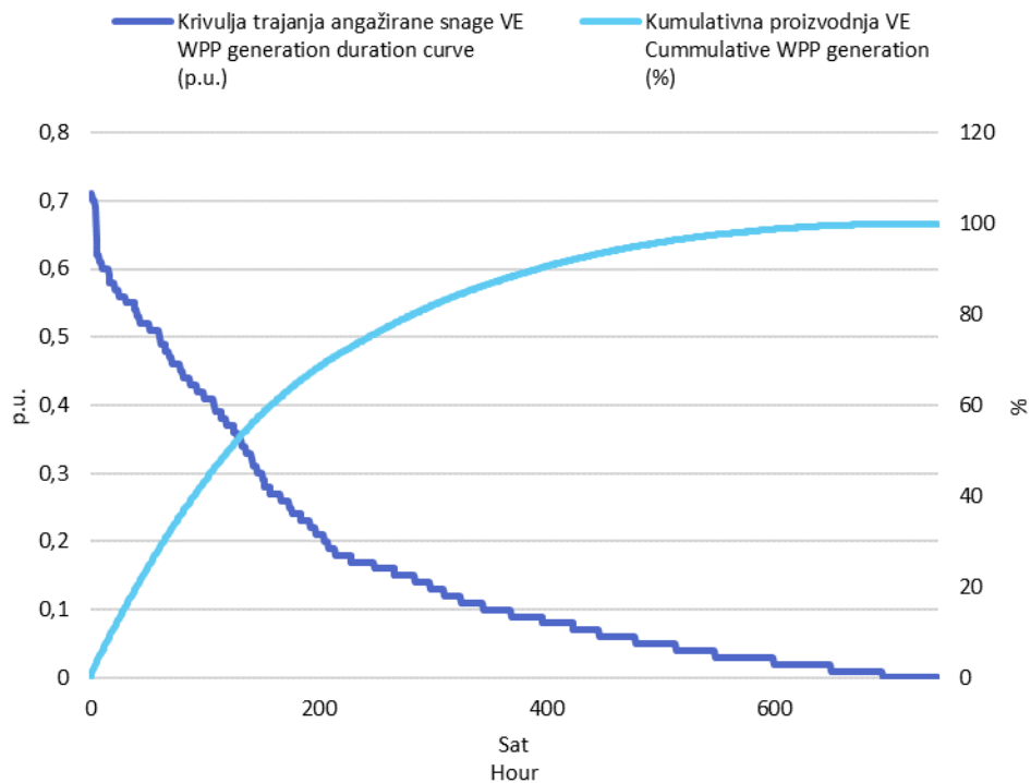
Slika 3 Krivulja trajanja angažirane snage svih VE i kumulativna proizvodnja VE u listopadu 2022. godine u jediničnim vrijednostima
