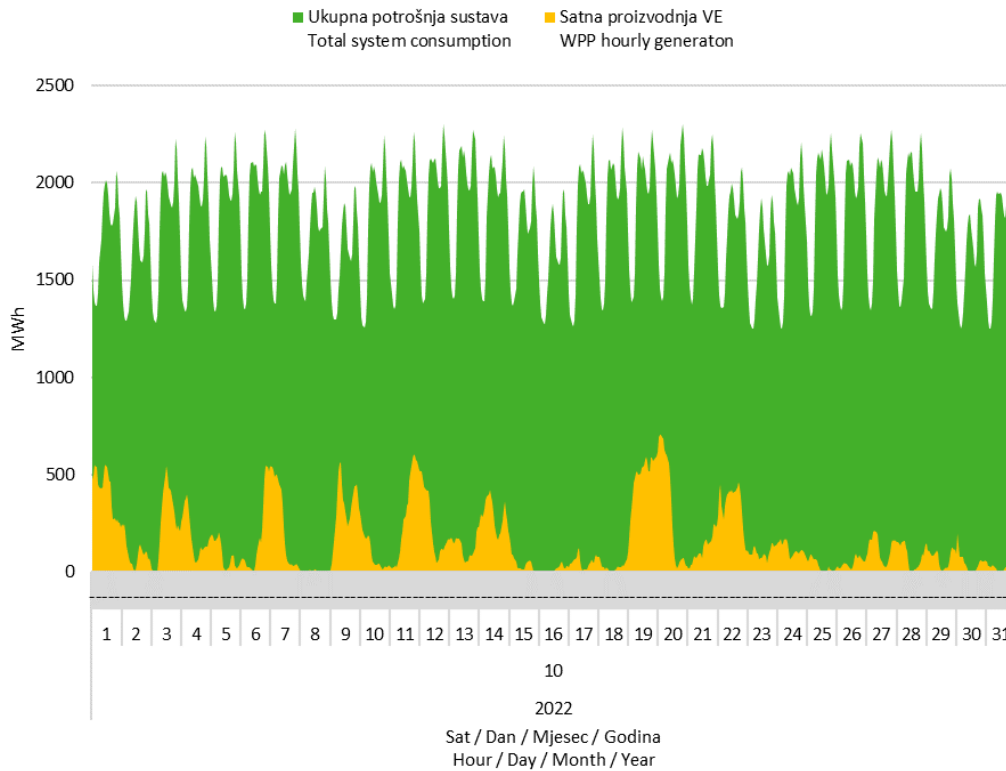
Slika 7 Usporedba satnog dijagrama opterećenja sustava i proizvodnje vjetroelektrana u listopadu 2022. godine
