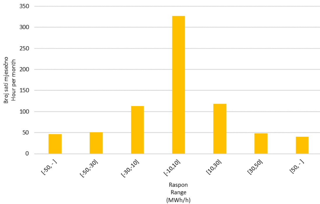
Slika 10 Statistička raspodjela satnih promjena proizvodnje VE u listopadu 2022. godine
