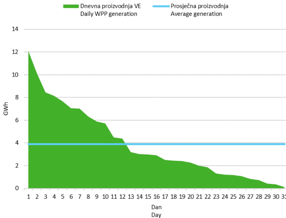
Slika 6 Krivulja trajanja dnevne proizvodnje vjetroelektrana u listopadu 2022. godine
